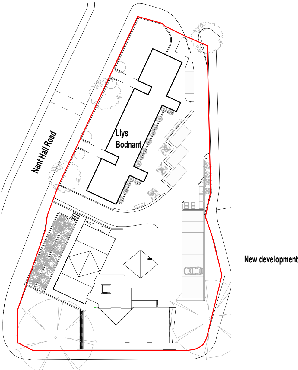
2 Site Block Plan 1 : 500
